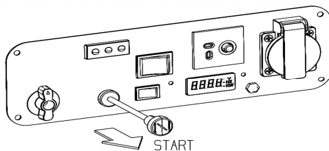
Abbildung 7. Starterklappe für Kaltstart aktiviert
