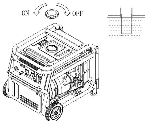
Ilustración 4. Diagrama de nivel de combustible
